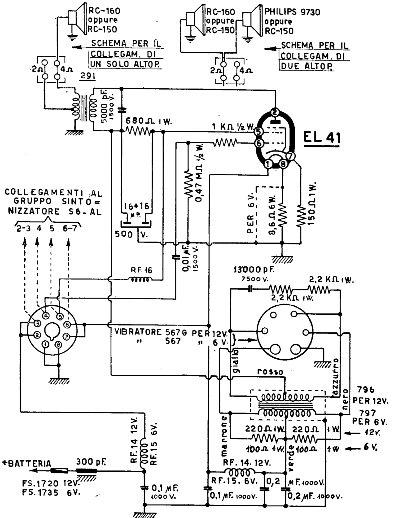
GALLO-CONDOR - Mod. S6 e S8. Unità alimentatrice e amplificatrice finale.
